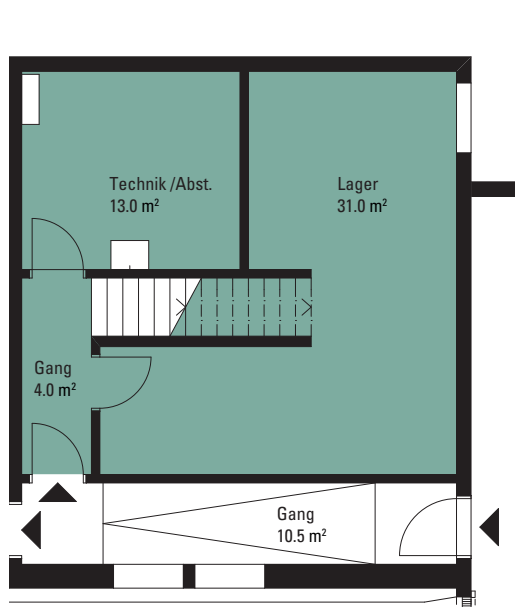
Untergeschoss
